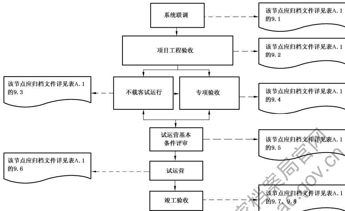
图4 项目竣工验收阶段关键环节及应归档文件
